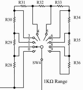
R28-R36 1K
