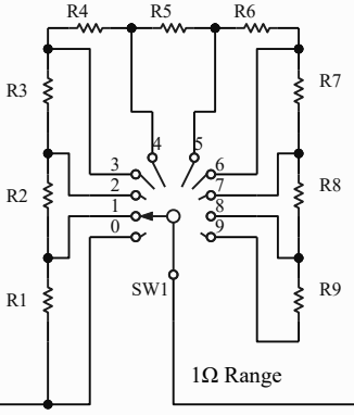
R1-R9 1R
