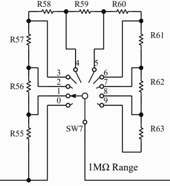
R55-R63 1M
